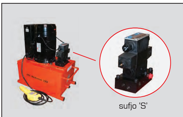
Válvula solenoide de baja tensión con control remoto manual y colgante
